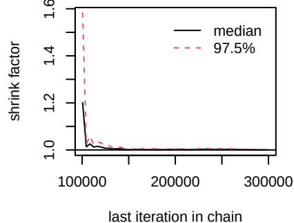
d.Osimertinib.Lazertinib_Amivanta
