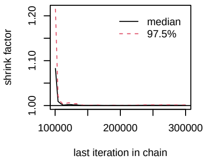
d.Osimertinib.Lazertinib
