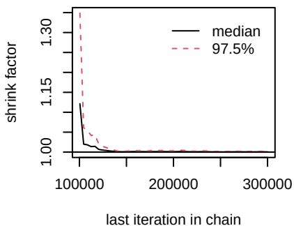
d.chemo.Erlotinib
