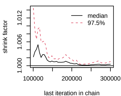
d.Erlotinib.antiangio
