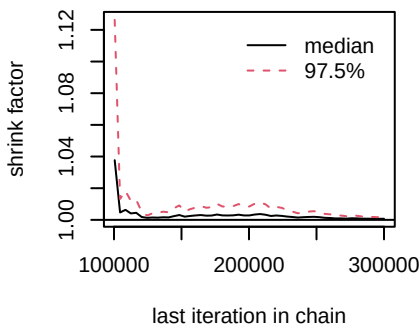
d.Gefitinib.Almonertinib
