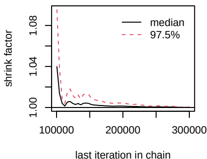
d.Gefitinib.Furmonertinib
