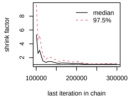
d.Erlotinib.Erlotinib_COX2i
