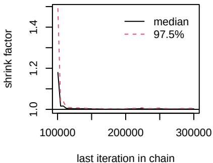
d.Afatinib.Afatinib_Cetuximab
