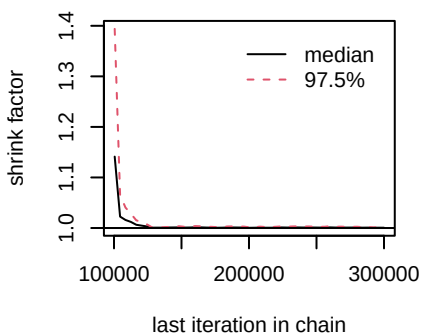
d.chemo.Osimertinib
